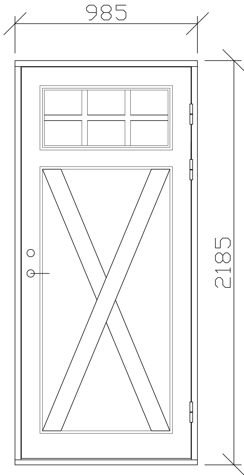
YD1 RMDÖRREN EY-SP BASIC, SLÄT INSIDA
